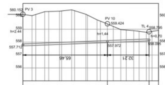
Perfil Longitudinal RUA 3 ( SUCATA)
