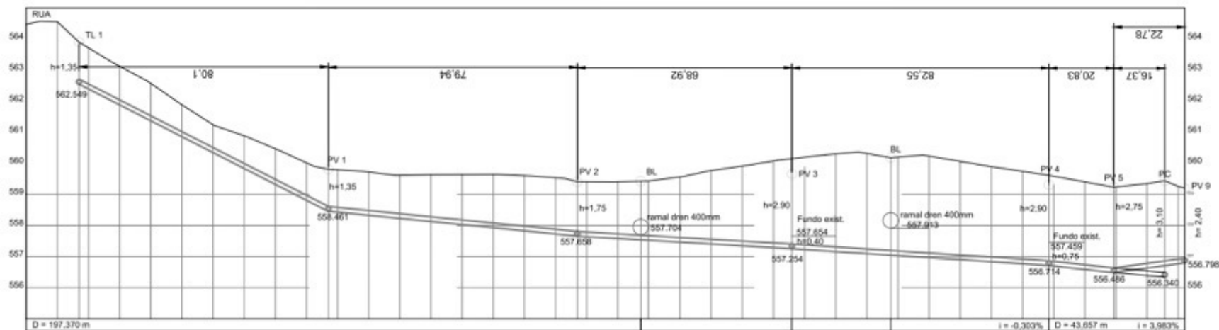
Perfil Longitudinal - RUA PAULO VELLOZO
