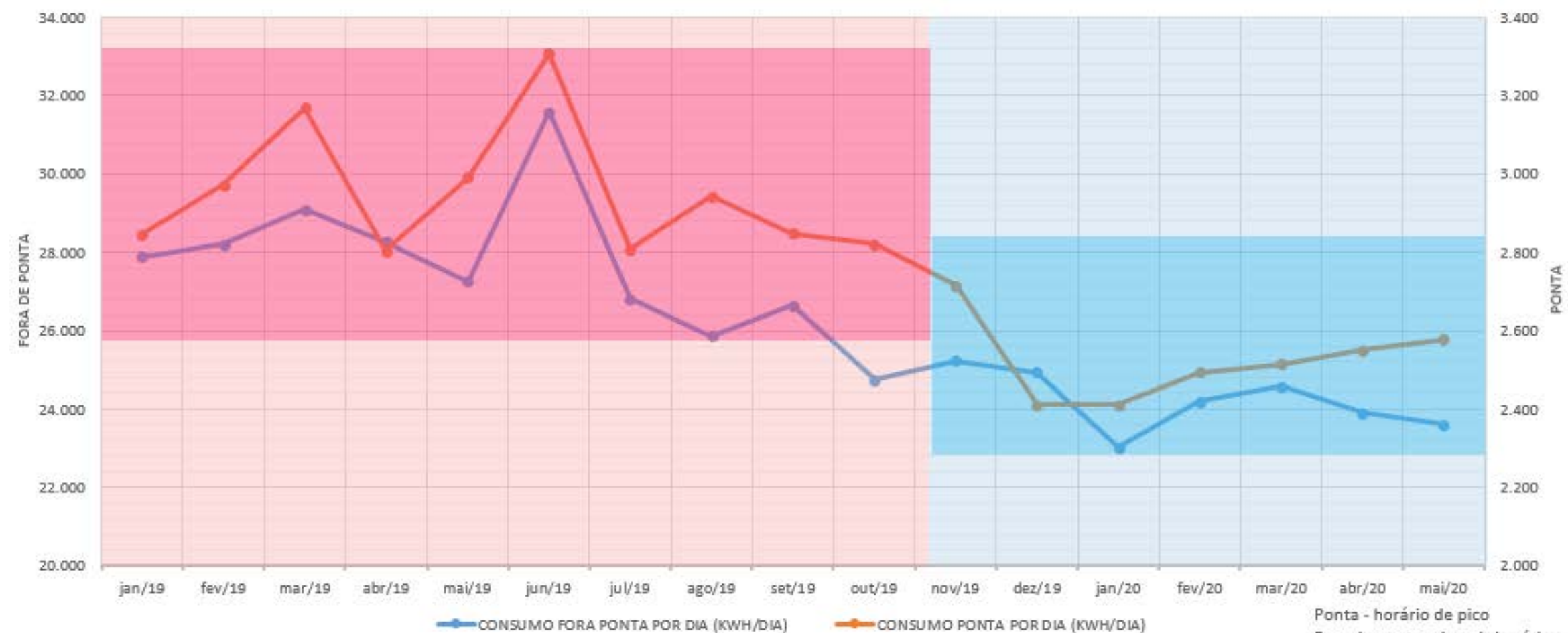
CONSUMO DE ENERGIA POR DIA - PONTA E FORA DE PONTA
