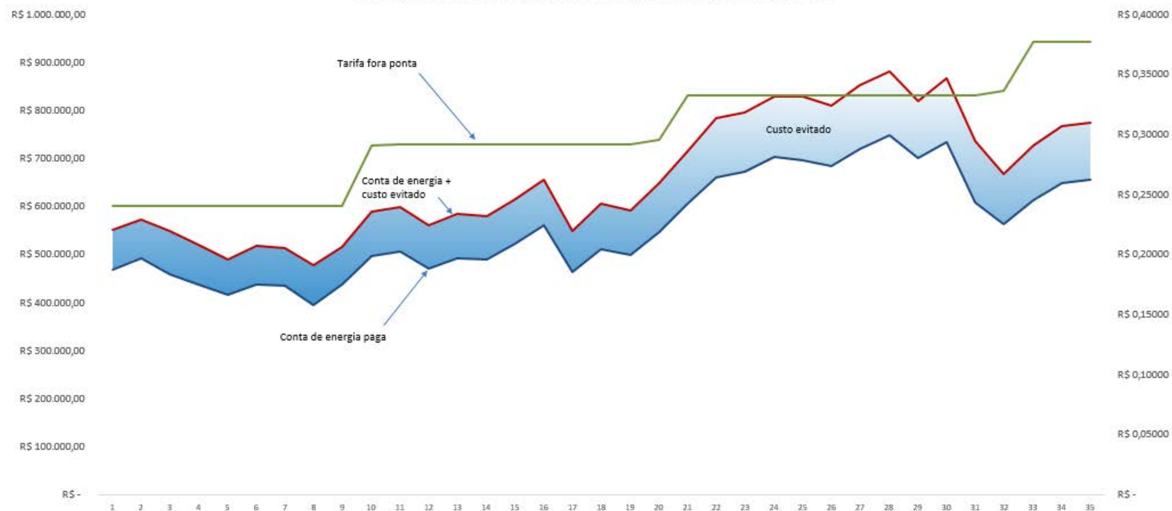
CONTA MENSAL DE ENERGIA, CUSTO EVITADO E TARIFA DE ENERGIA
