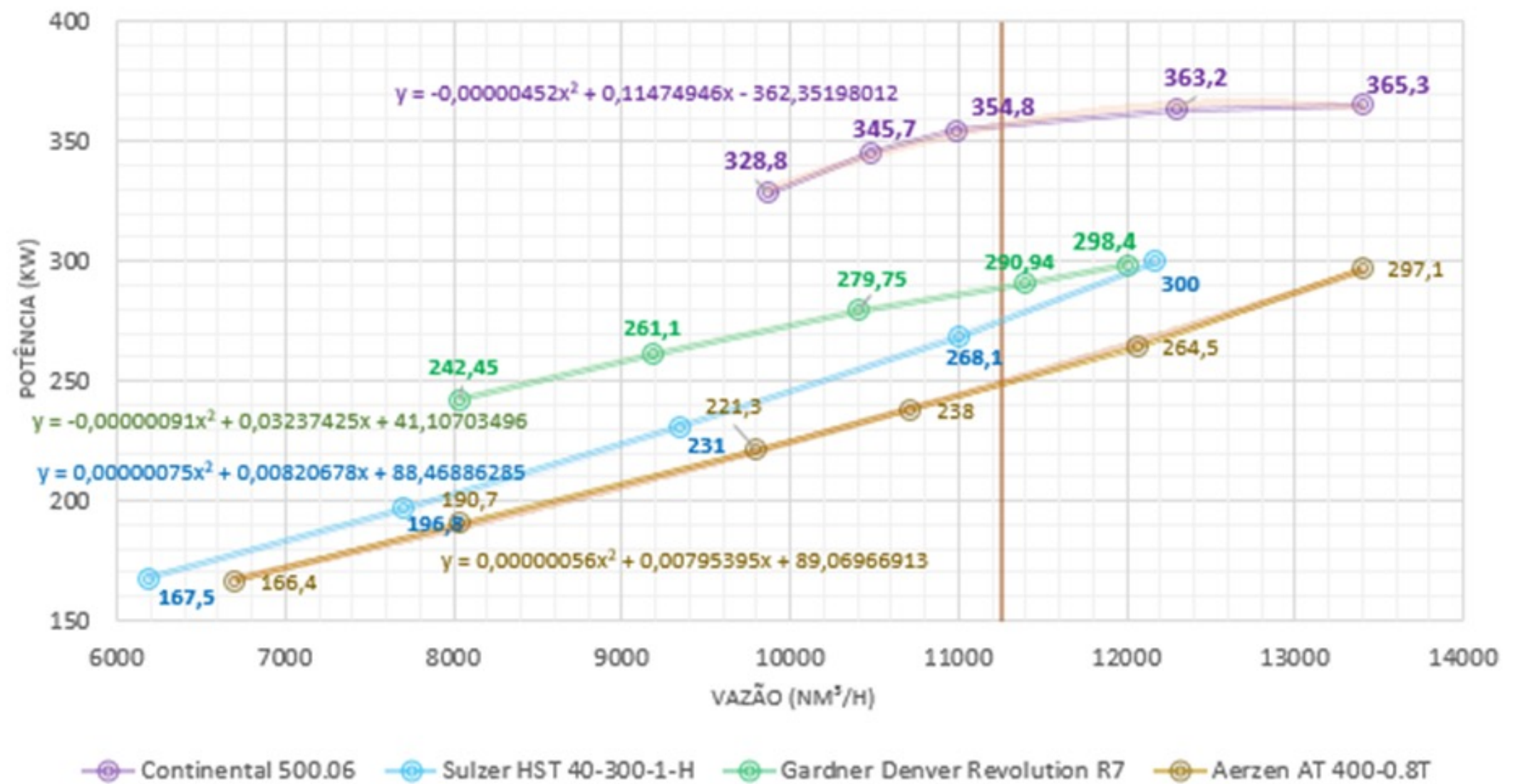
Potência x Vazão
